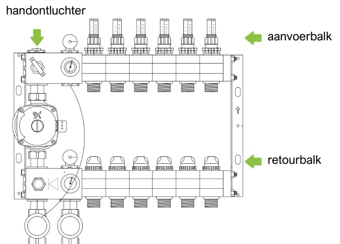
Topline SV-verdeler met onderaansluiting
