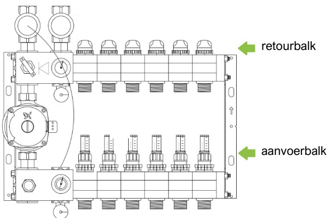
Topline SV-verdeler met bovenaansluiting
